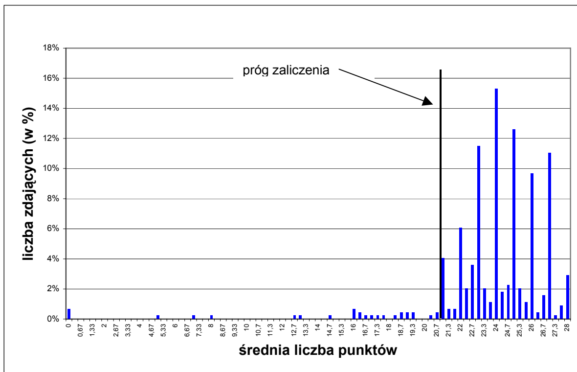
Wykres 4. Rozkład wyników etapu praktycznego dla zawodu operator obrabiarek skrawających w skali kraju
