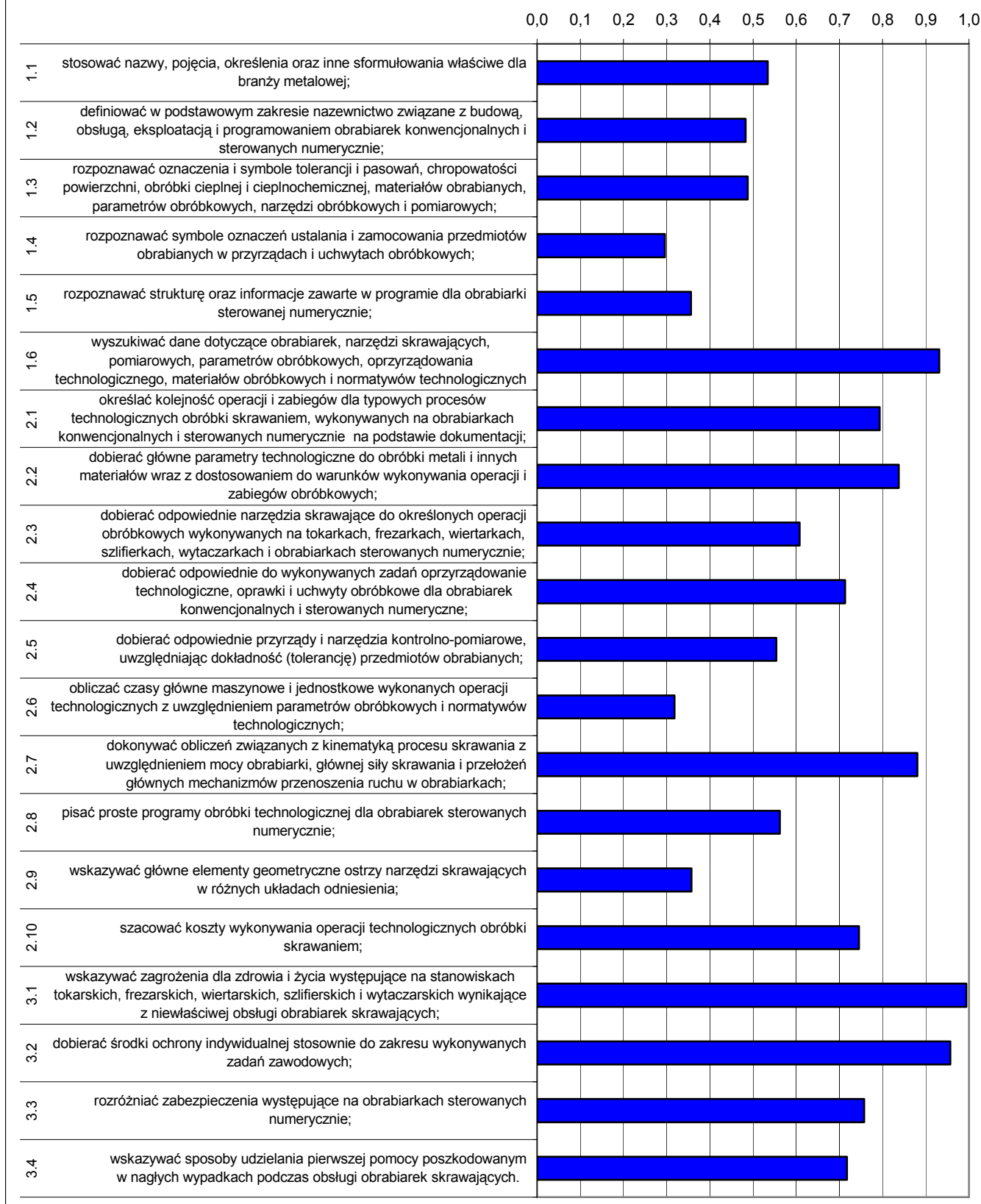
Wykres 3. Średnia łatwość umiejętności sprawdzanych w części I etapu pisemnego dla zawodu operator obrabiarek skrawających
