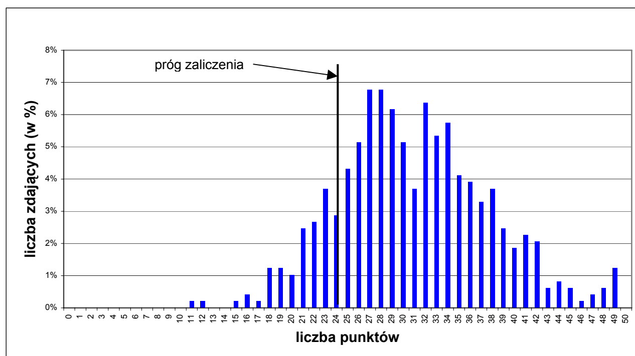
Wykres 1. Rozkład wyników części I etapu pisemnego dla zawodu operator obrabiarek skrawających w skali kraju
