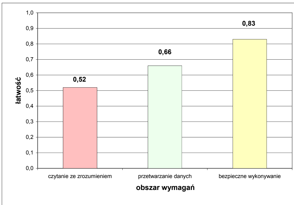
Wykres 2. Średnia łatwość zadań w obszarach części I etapu pisemnego dla zawodu operator obrabiarek skrawających
